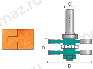
3523 Фреза комбинированная паз-шип
