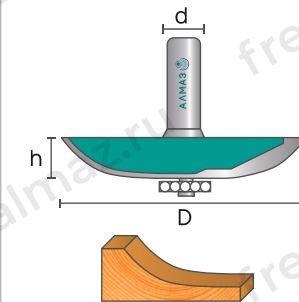
3001 Фреза фигурейная горизонтальная
