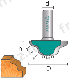
2030 Фреза кромочная калёвочная
