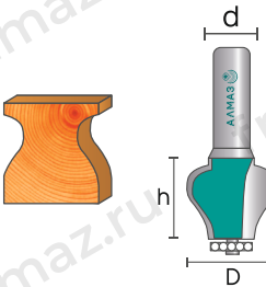
2205 Фреза кромочная фигурейная
