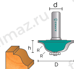
2004 Фреза кромочная калёвочная
