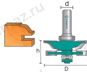
3504 Фреза комбинированная рамочная
