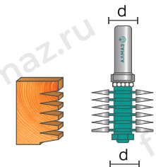
2550 Фреза микрошип
