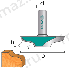
2155 Фреза фигурейная горизонтальная
