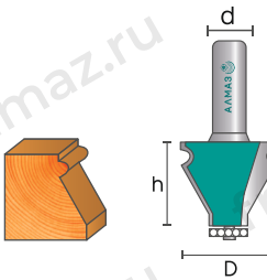
2217 Фреза кромочная фигурейная
