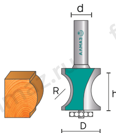
1013 Фреза кромочная полустержневая
