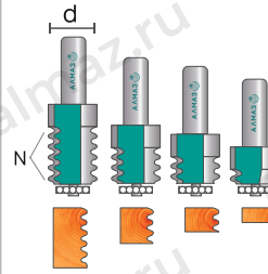
2600 Фреза микрошип
