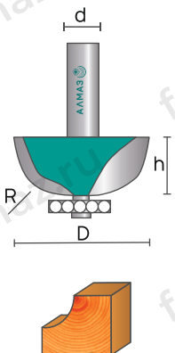
1018 Фреза кромочная калёвочная
