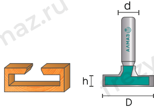
2511 Фреза конструкционная Т-обр.
