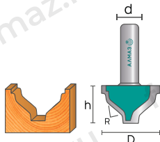
2056 Фреза пазовая фасонная
