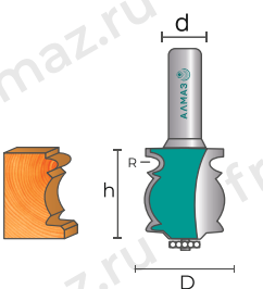
2038 Фреза кромочная фигурная
