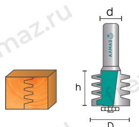
2501 Фреза микрошип
