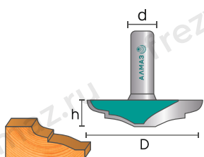
2402 Фреза пазовая фасонная
