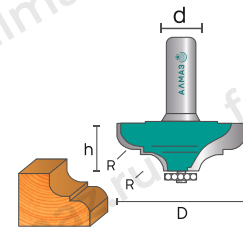
2002 Фреза кромочная калёвочная
