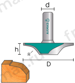
2156 Фреза фигурейная горизонтальная
