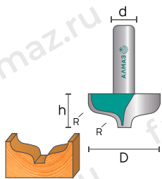
2055 Фреза пазовая фасонная
