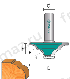
2009 Фреза кромочная калёвочная
