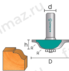
2104 Фреза фигурная горизонтальная
