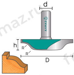
2154 Фреза фигурейная горизонтальная
