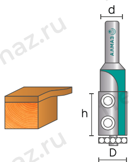
120 Фреза со сменными пластинами кромочная прямая
