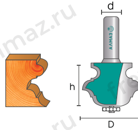
2040 Фреза кромочная мультипрофильная
