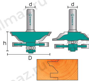
3504 set Фреза рамочная
