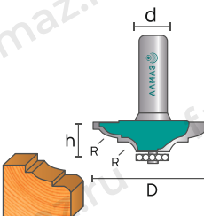
2103 Фреза фигурная горизонтальная
