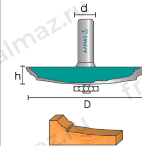
3002 Фреза фигурейная горизонтальная
