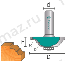
2101 Фреза фигурная горизонтальная
