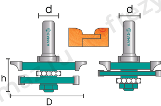
3551 set Фреза для изготовления вагонки
