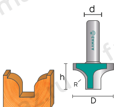
2057 Фреза пазовая фасонная
