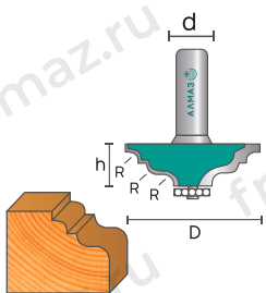
2011 Фреза кромочная калёвочная
