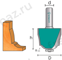
3012 Фреза фигурейная вертикальная
