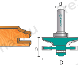
3502 Фреза комбинированная рамочная
