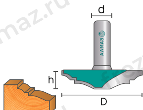
2412 Фреза пазовая фасонная
