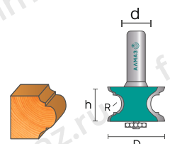
2015 Фреза кромочная фигурная
