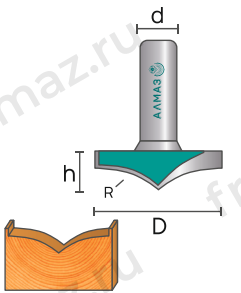
2157 Фреза фигурейная горизонтальная
