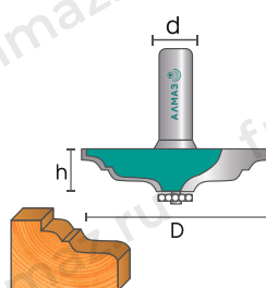
2111 Фреза фигурная горизонтальная
