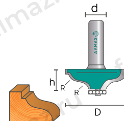
2006 Фреза кромочная калёвочная
