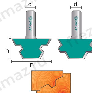
3510 set Фреза для срашивания
