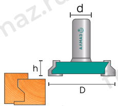
2512 Фреза пазовая конструкционная Т-обр.
