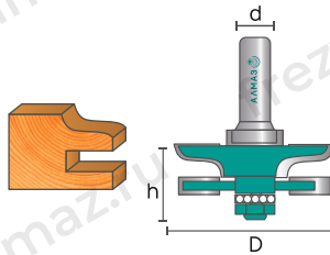
3505 Фреза комбинированная рамочная
