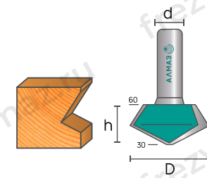
2516 Фреза кромочная конусная
