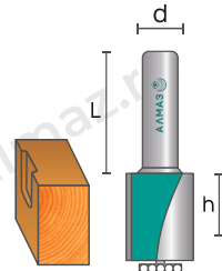
1120 Фреза кромочная прямая
