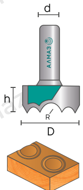
1027 Фреза фасонная
