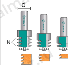
2601 Фреза микрошип
