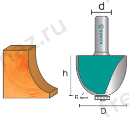
3011 Фреза фигурейная вертикальная
