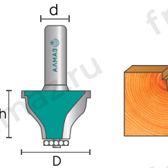
2206 Фреза кромочная фигурейная
