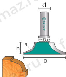
2307 Фреза кромочная калёвочная
