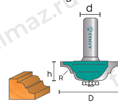
2001 Фреза кромочная калёвочная
