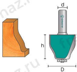
3013 Фреза фигурейная вертикальная
