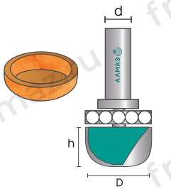
2166 Фреза пазовая фасонная для изготовления чаш, менажниц
