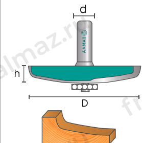
3005 Фреза фигурейная горизонтальная
