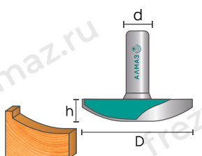
2405 Фреза пазовая фасонная
