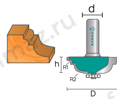
2021 Фреза кромочная калёвочная
