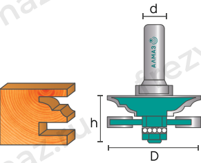
3501 Фреза комбинированная рамочная
