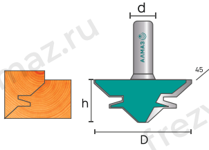
2510 Фреза комбинированная универсальная
