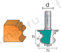
2020 Фреза кромочная мультипрофильная
