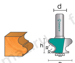
2019 Фреза кромочная мультипрофильная
