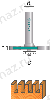
1023 z3 Фреза кромочная фальцевая
