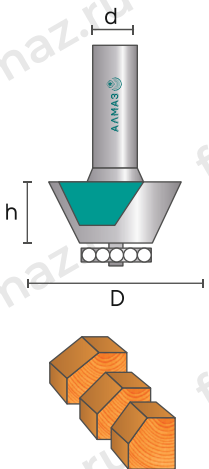
1024 Фреза кромочная конусна
