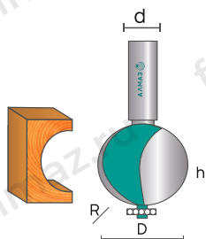
1015 Фреза кромочная галтельная
