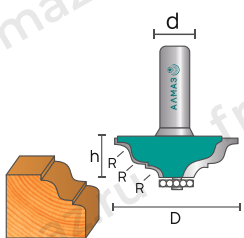
2012 Фреза кромочная калёвочная
