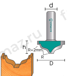
2059 Фреза пазовая фасонная
