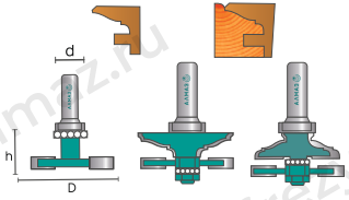
3512 set Набор рамочных фрез
