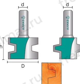
3511 set Фреза паз-шип
