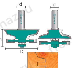
3502 set Фреза рамочная
