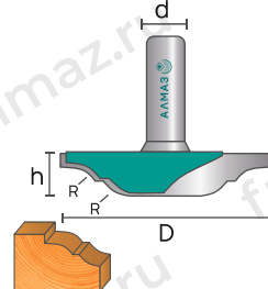
2151 Фреза фигурная горизонтальная
