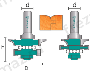
3550 set Фреза для изготовления вагонки
