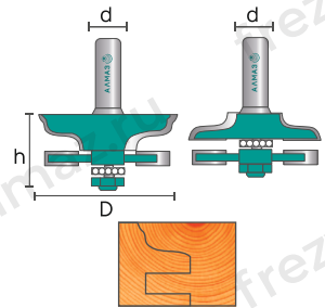
3505 set Фреза рамочная
