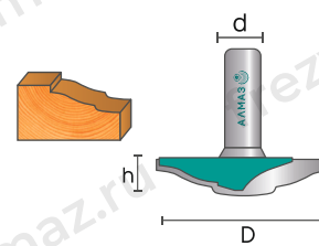
2416 Фреза пазовая фасонная
