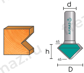
2515 Фреза кромочная конусная
