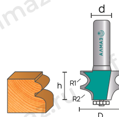
2025 Фреза кромочная фигурная
