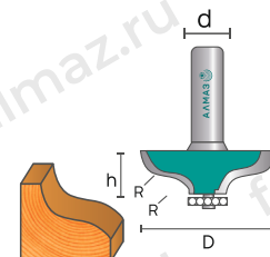
2005 Фреза кромочная калёвочная
