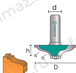
2106 Фреза фигурная горизонтальная
