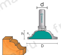
2301 Фреза кромочная калёвочная
