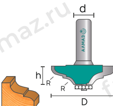
2102 Фреза фигурная горизонтальная
