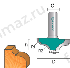
2022 Фреза кромочная калёвочная
