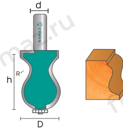
2204 Фреза кромочная фигурейная
