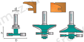
3515 set Набор рамочных фрез
