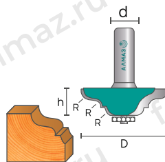
2014 Фреза кромочная калёвочная
