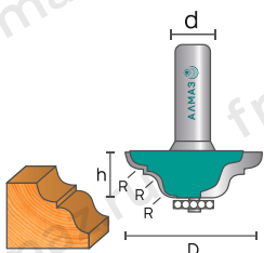
2013 Фреза кромочная калёвочная
