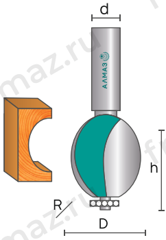
1016 Фреза кромочная галтельная
