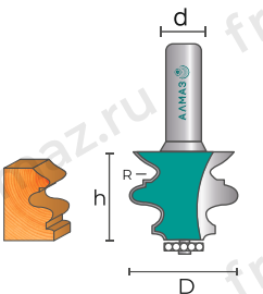
2037 Фреза кромочная фигурная
