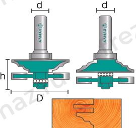
3501 set Фреза рамочная
