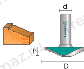
2433 Фреза пазовая фасонная
