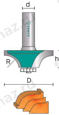
1019 Фреза кромочная калёвочная
