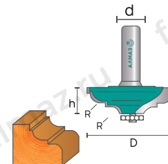
2003 Фреза кромочная калёвочная
