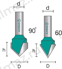
1004 Фреза пазовая галтельная V-form
