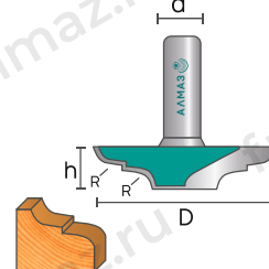
2152 Фреза фигурная горизонтальная
